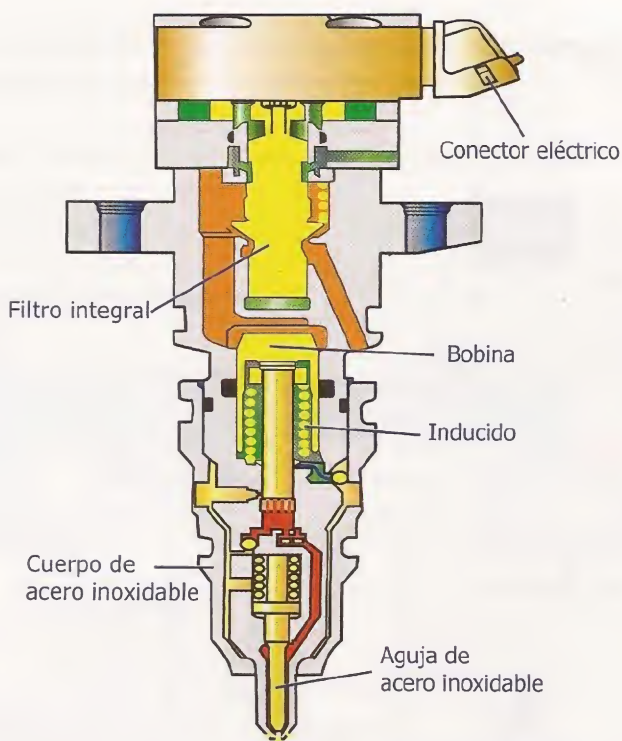
Inyector electrónico
